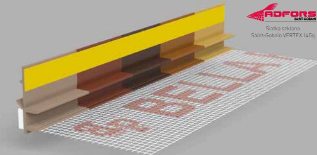
BP13 KOLOR 9/6 LISTWY PRZYOKIENNE KOLOROWE PVC DYLATACYJNE Z SIATKĄ I Z USZCZELKĄ 9mm (szerokość listwy) / 6mm (szerokość korytka)
